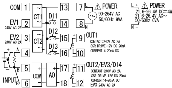
MAC 3 D端子配置圖
