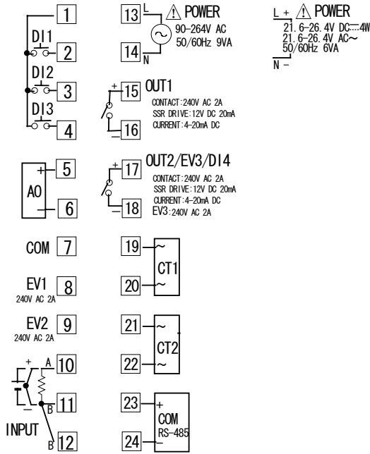
MAC 3 A & MAC 3 B 端子配置圖
