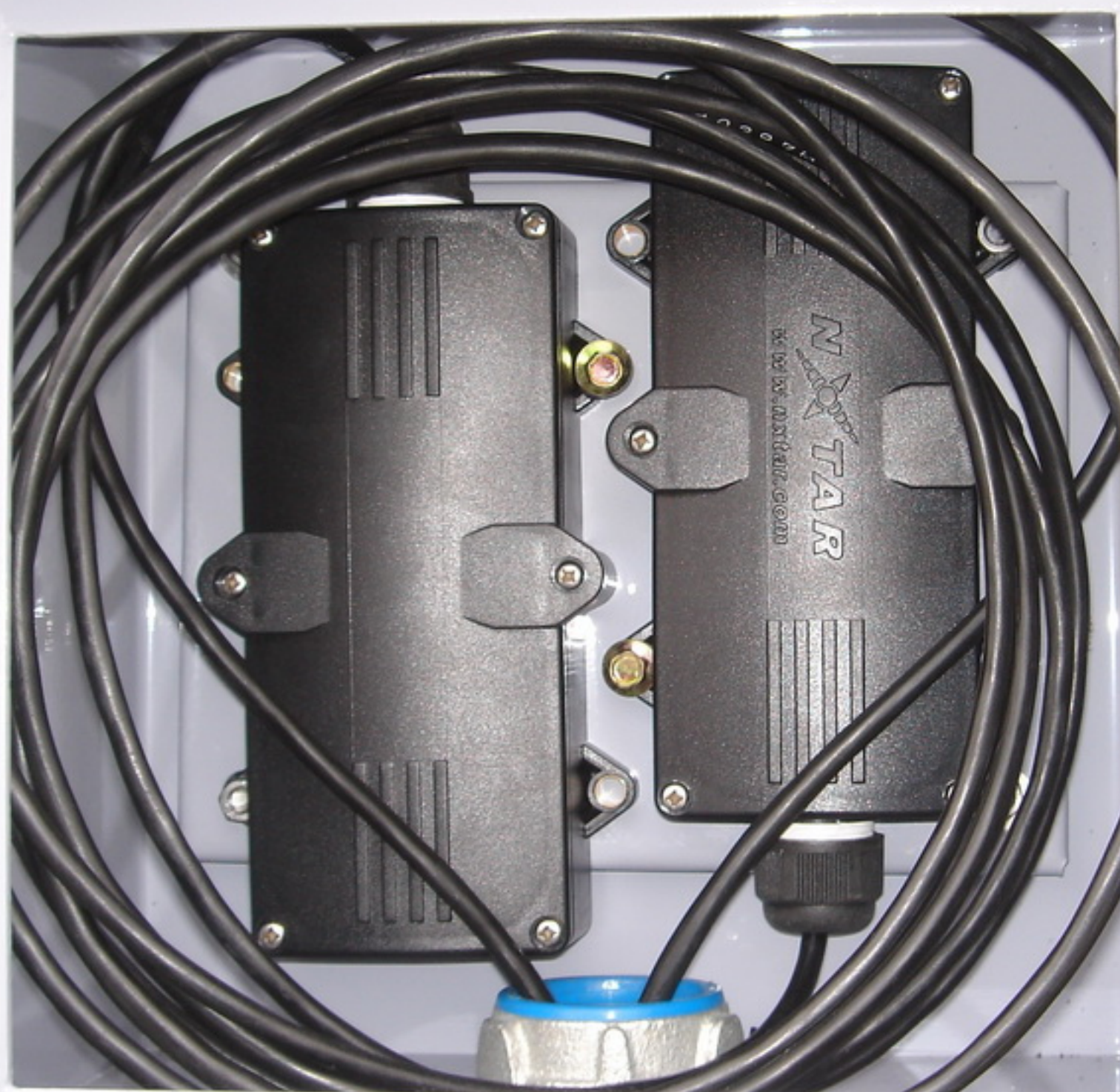
相鄰兩區的TJB，共用同一防水箱。
