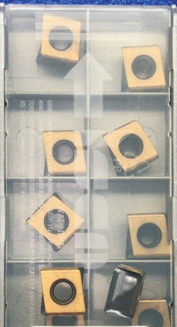
AREFU 新品 日本外匯 新品 刀片 伊斯卡 ISCAR LNHT 1006 ER IC810
