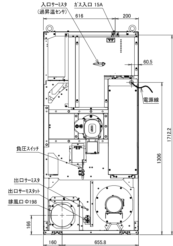
VG143外觀図
